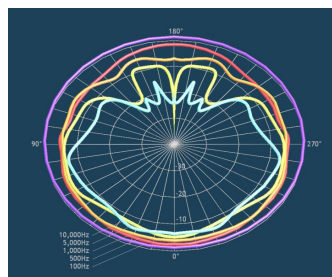
一般的なスピーカーの指向特性
